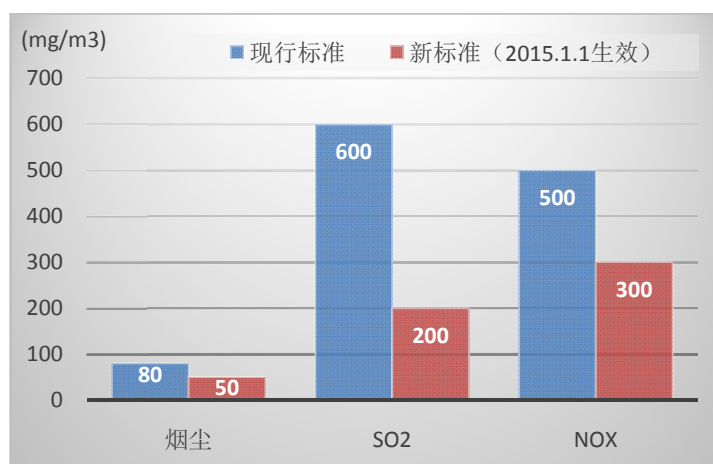
图 32 《钢铁烧结、球团工业大气污染物排放标准》比较 19
