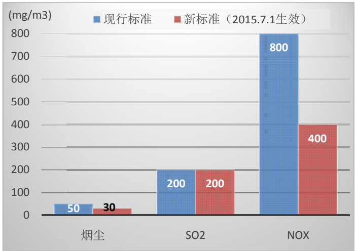
图 34 《水泥工业大气污染物排放标准》比较 21
