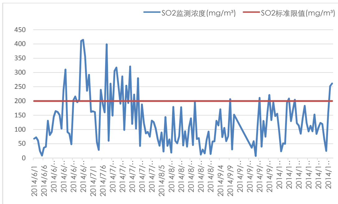
图 8 临澧冀东水泥有限公司回转窑排口二氧化硫日均值浓度 (时间: 2014 年 6-10 月)
