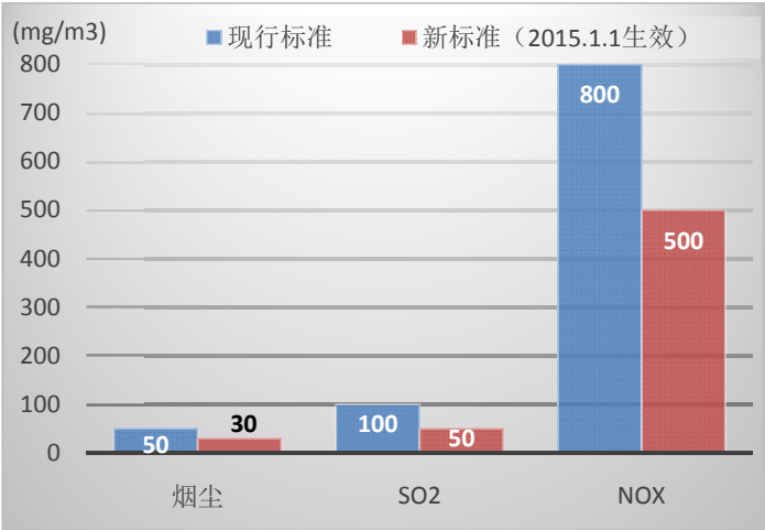
图 33 《炼焦化学工业污染物排放标准》比较 20
