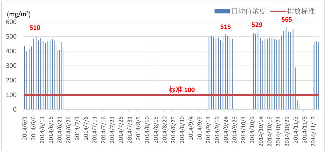
图 11 中国铝业股份有限公司山东分公司热电厂/中铝热电（1-2）氮氧化物日均值浓度（2014 年 6-11 月）
