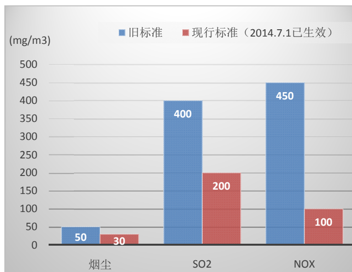
图 31 《火电厂大气污染物排放标准》比较 18
