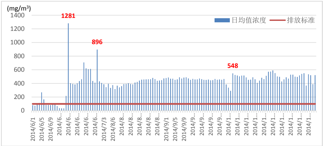
图 12 中国铝业股份有限公司山东分公司热电厂/中铝热电（3）氮氧化物日均值浓度（2014 年 6-11 月）
