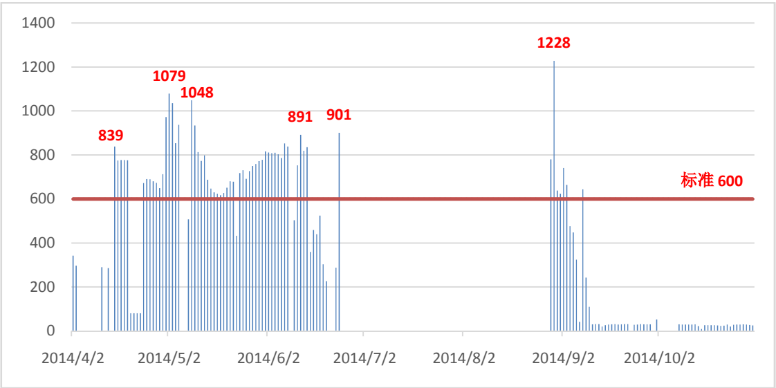
图 20 湖南华菱涟源钢铁有限公司 360 机头二氧化硫日均值监测浓度（2014 年 4 月-10 月）
