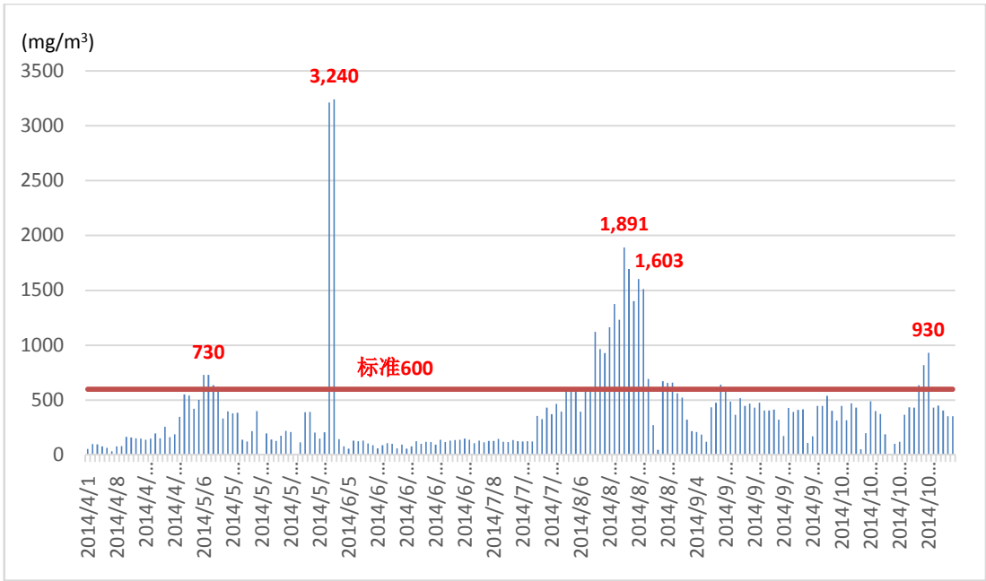
图 15 内蒙古包钢钢联股份有限公司炼铁厂四烧二期烧结机机头二氧化硫日均值监测浓度（2014 年 4-10 月）
