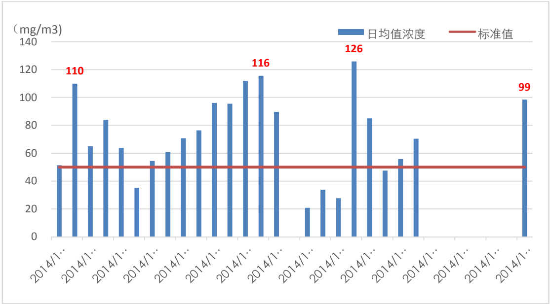
图9 冀东水泥磐石有限责任公司 2014 年 10 月，排口 2 号窑尾烟尘日均浓度值
