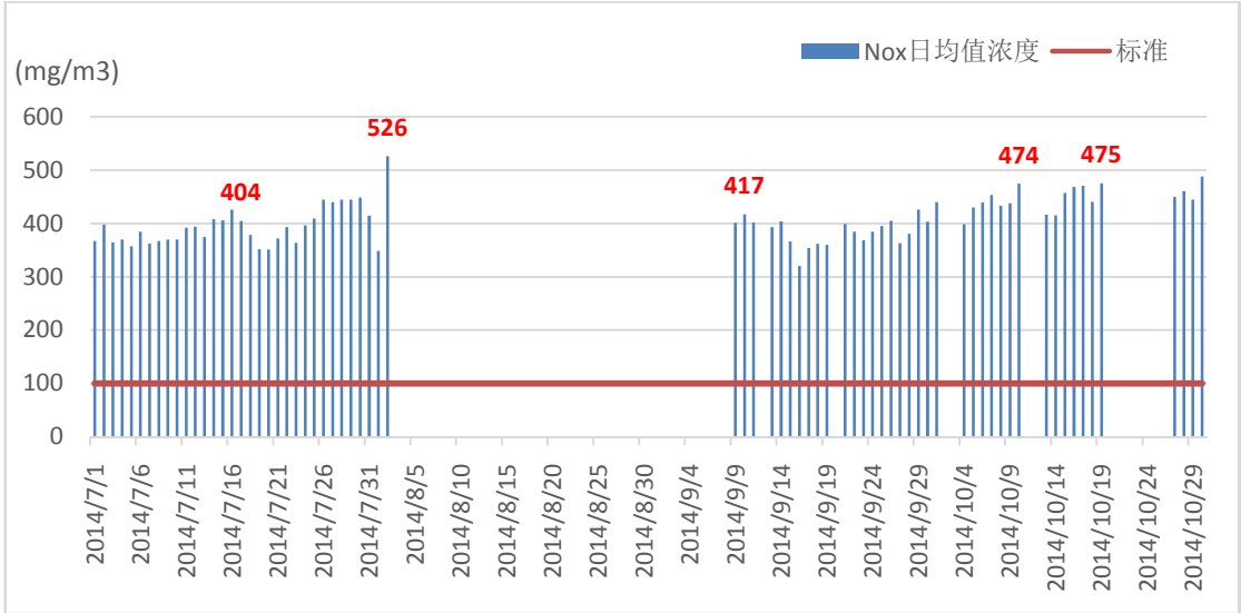
图 17 内蒙古包钢钢联股份有限公司热电厂 2#脱硫系统出口烟气氮氧化物在线监测浓度（2014 年 7-10 月）
