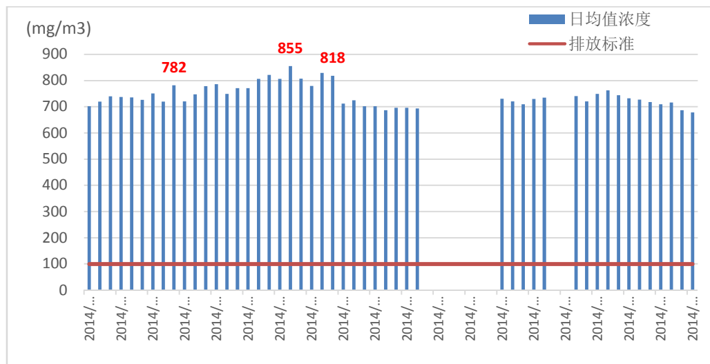
图 13 中国铝业股份有限公司中州分公司 1#-3#热电厂锅炉氮氧化物日均值浓度 (2014.9-11 月)
