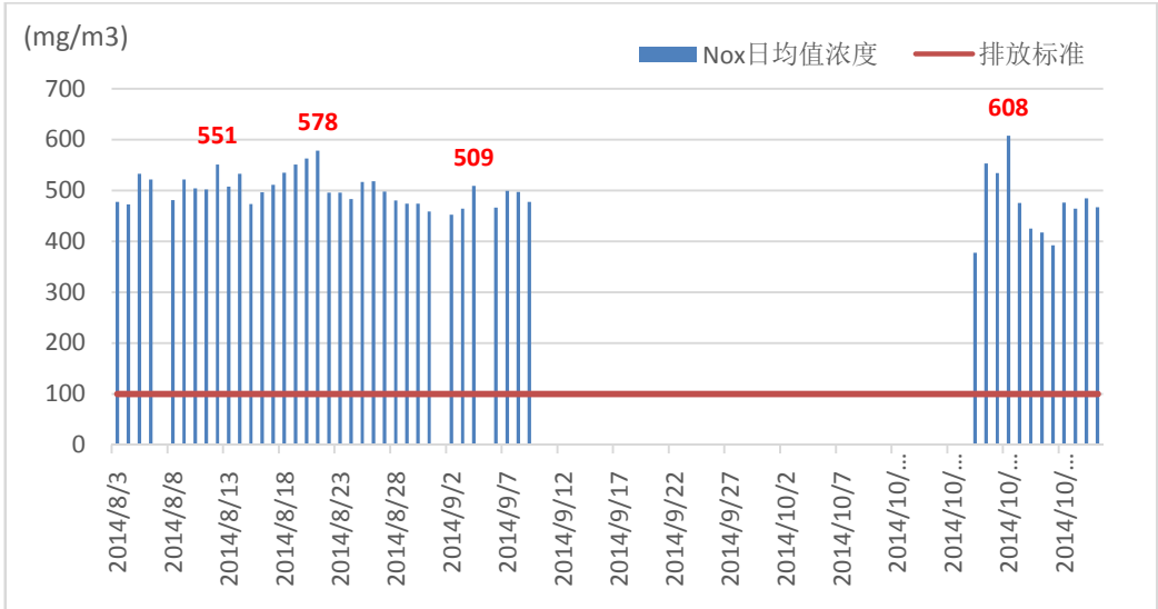
图 16 内蒙古包钢钢联股份有限公司热电厂 1#脱硫系统出口烟气氮氧化物在线监测浓度（2014 年 8-10 月）
