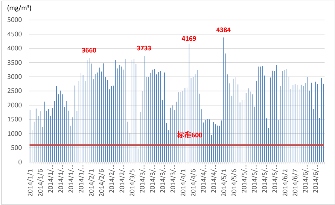
图 14 内蒙古包钢钢联股份有限公司炼铁厂三烧烧结机机头二氧化硫日均值监测浓度（2014 年 1-6 月）
