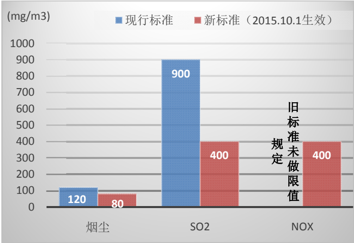
图 35 《锅炉大气污染物排放标准》比较 22
