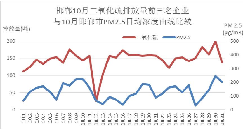
图 40 邯郸 10 月二氧化硫排放量前三名企业与 PM 2.5 日均浓度曲线对比
