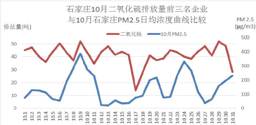
图 41 石家庄 10 月二氧化硫排放量前三名企业与 PM 2.5 日均浓度曲线对比
