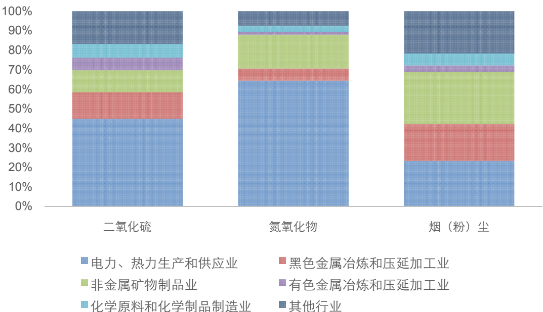
图 2 五个重点工业行业排放大气污染物占比（来源：2012 年中国环境统计公报）
