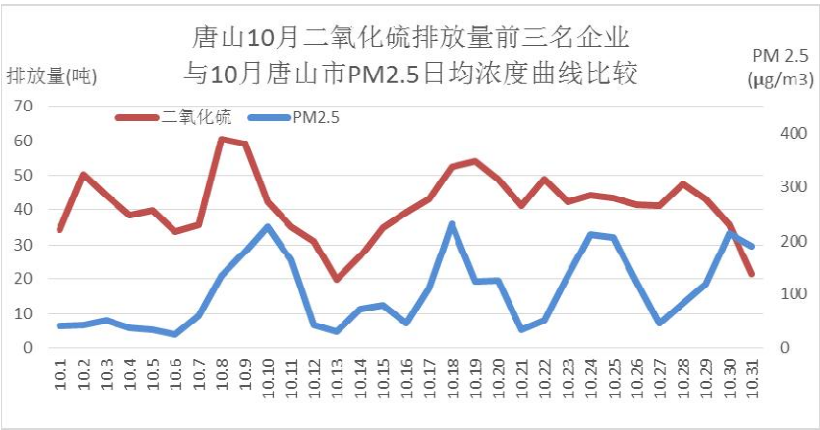
图 39 唐山 10 月二氧化硫排放量前三名企业与 PM 2.5 日均浓度曲线对比
